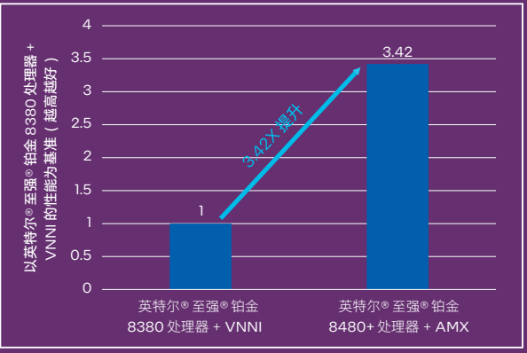
图 2. 第三代/第四代英特尔® 至强® 可扩展处理器 OCR 算法推理性能对比 (时延 <30ms)
